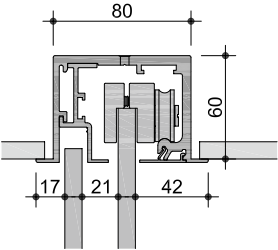
Pareti scorrevoli - Scorrimento interno vano Sliding doors - Internal
