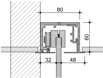
Porte scorrevoli - Scorrimento esterno vano Sliding doors - External
