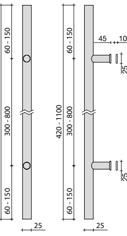
Maniglione singolo altezza mm 420/1100 Single pullhandle height 420/1100 mm
