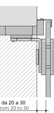
Fissaggio a parete Wall installation
