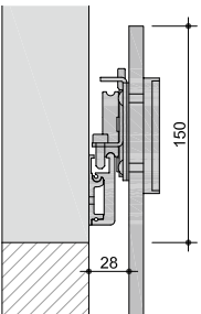
Porte scorrevoli Scorrimento esterno vano Sliding doors - External
