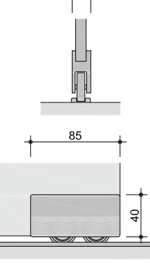
Particolare ruota Trolley detail
