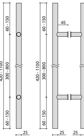
Maniglione doppio altezza mm 420/1100 Double pullhandle height 420/1100 mm
