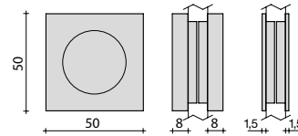
Maniglia quadrata ad incasso Escluso Synthesy Stylo e Quadra Recessed square handle Not available on Synthesy Stylo e Quadra
