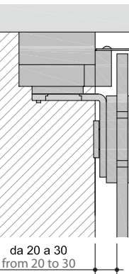
Fissaggio a soffitto Ceiling installation
